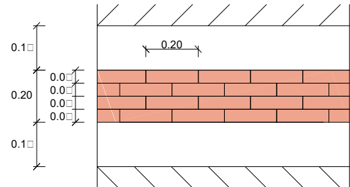
Planta col·locació paviment Stradalit ESCALA 1:20
