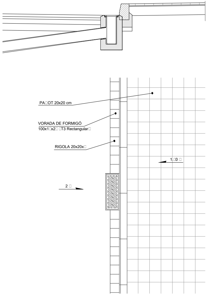
Detall paviment ESCALA 1:10
