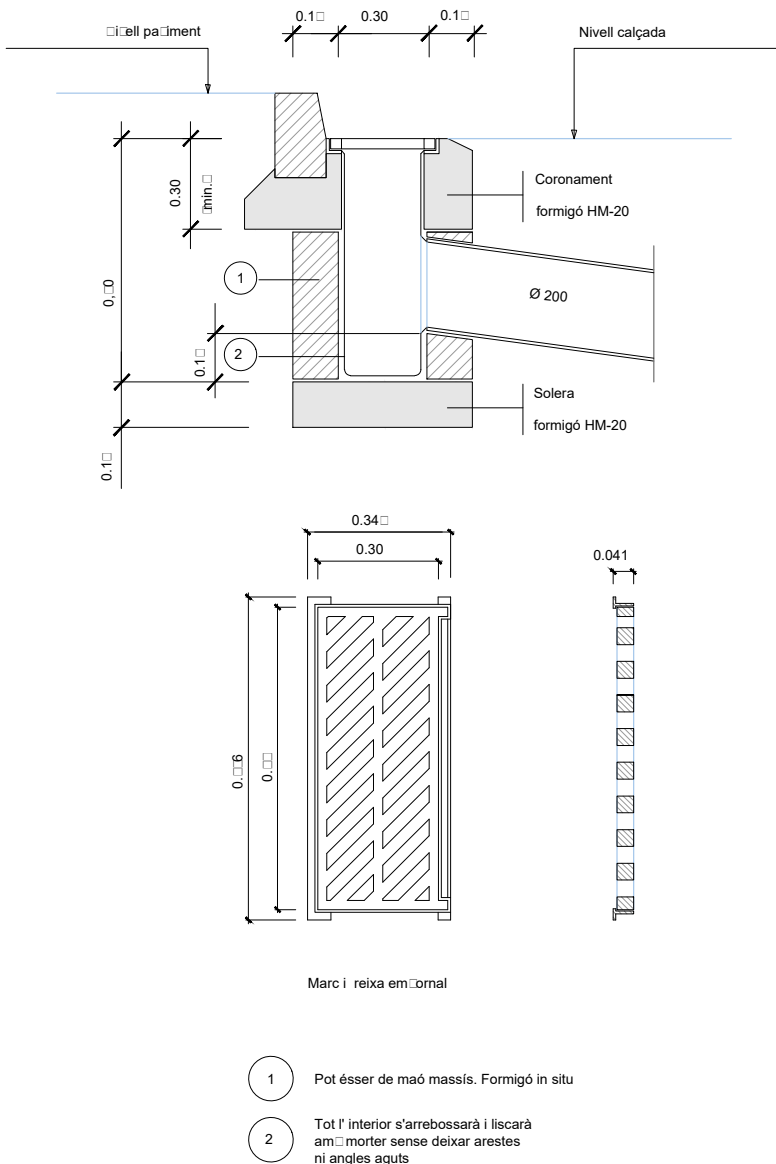
Detall emfornal xarxa pluvials ESCALA 1:2
