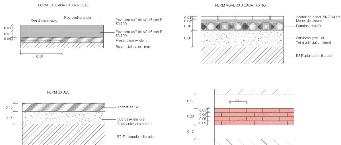
Detalls constructius de les tipologies de paviments
